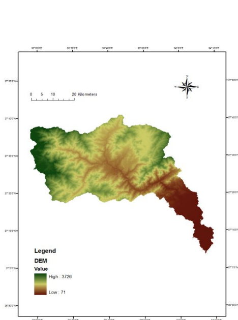
Figure 2: Ranganadi DEM
