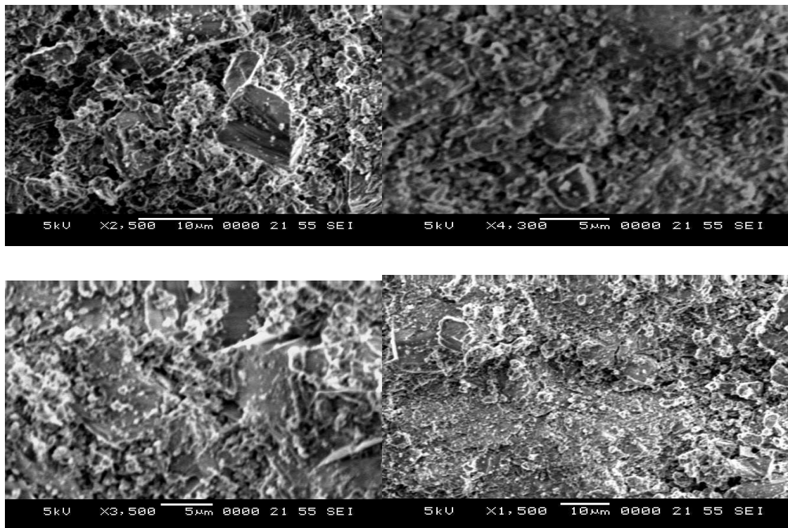
Fig. 2: SEM images of M 60 0% RHA
