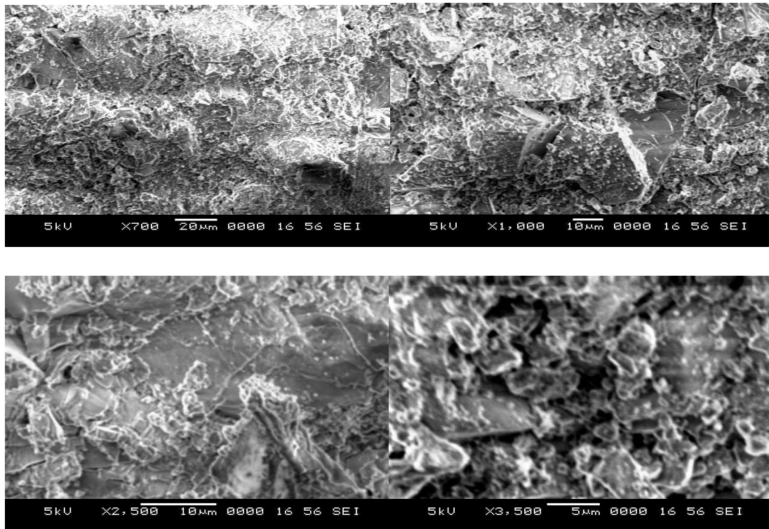
Fig. 3: SEM images of M 60 15% RHA.
