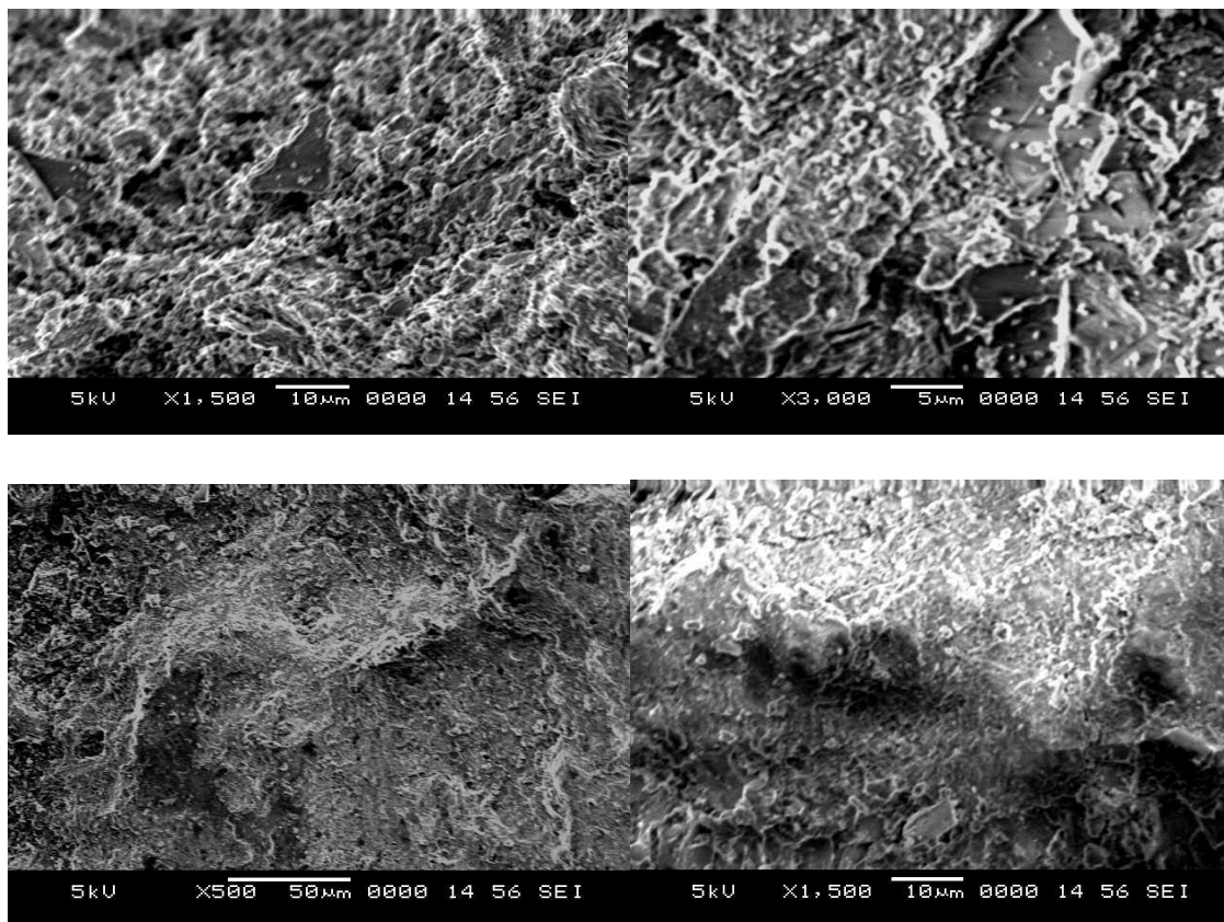
Fig. 5: SEM images of M 80 15% RHA.
