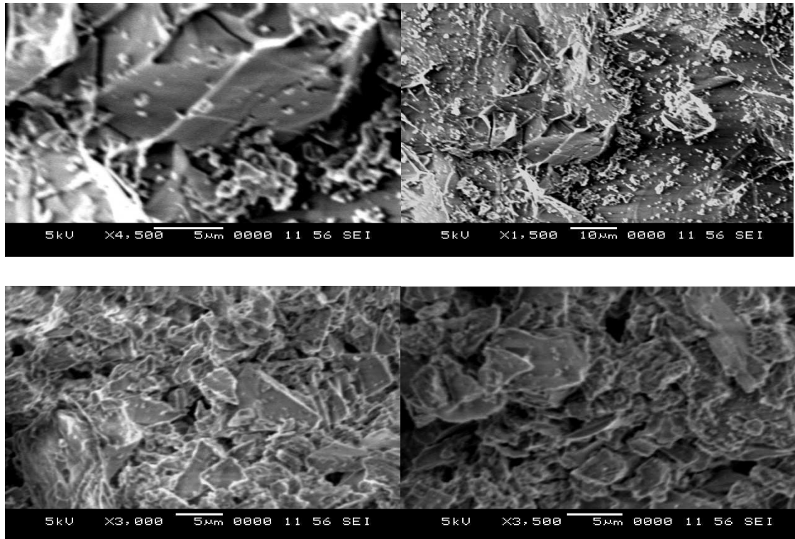
Fig. 7: SEM images of M 100 15% RHA.
